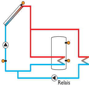
Variante Pumpe
