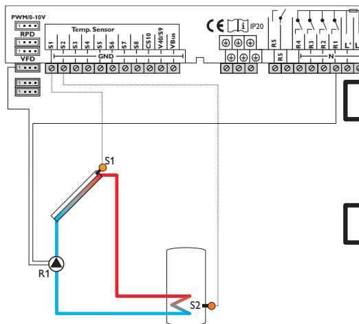
Beispiel für den elektrischen Anschluss einer Hocheffizienzpumpe
